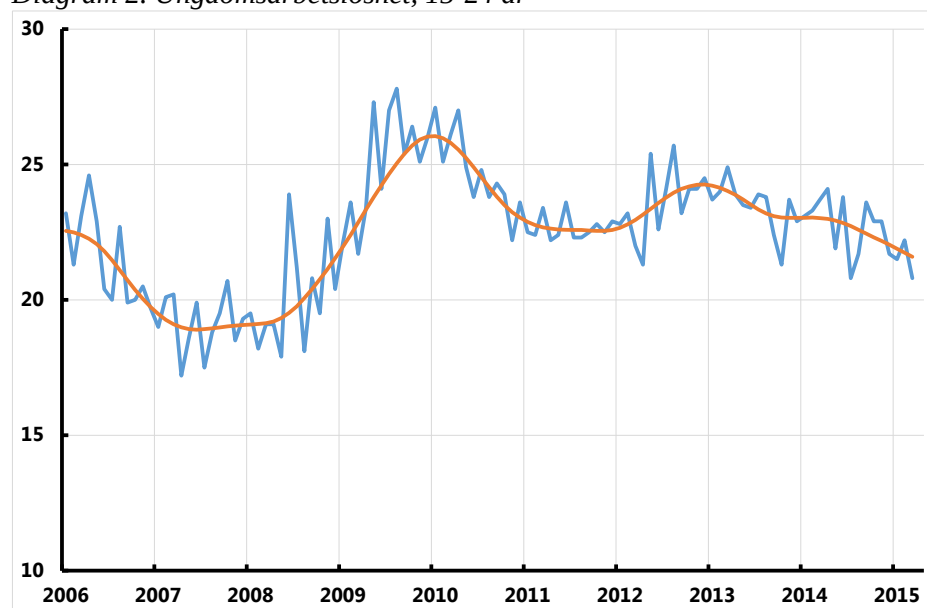
Diagram 2. Ungdomsarbetslöshet, 15-24 år
