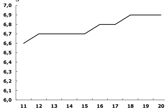
Diagram 2. Jämviktsarbetslöshet 2011–2020
